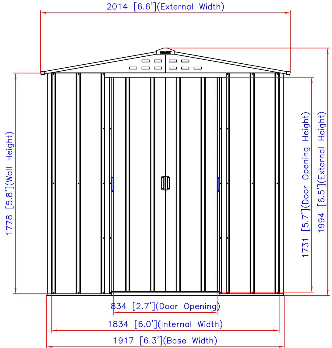
Elevation
